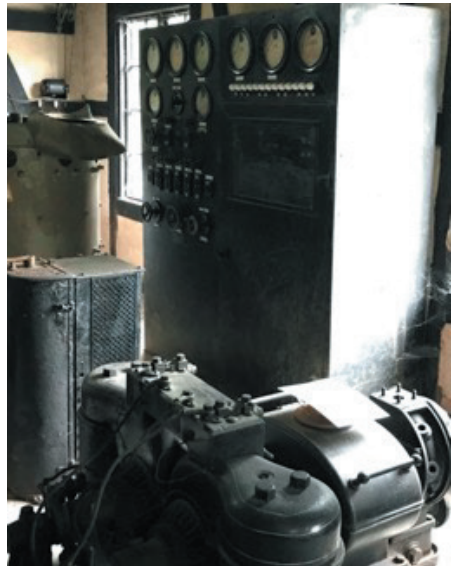
Ångturbindriven dubbelgenerator tillverkad i mitten av 1890-talet, utkast av Gustav de Laval, gav 20 hk (kunde få 240 s 25 Watts-lampor att lysa samtidigt).
